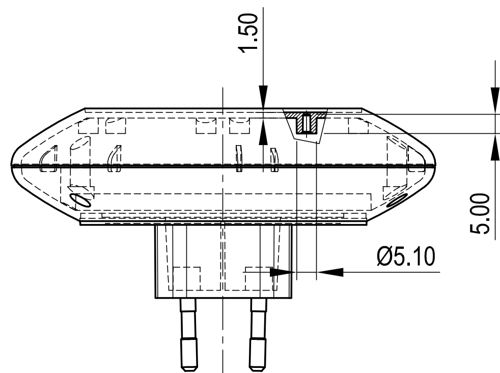
Unterteil- Innenansicht Bottom-Part Inside View
