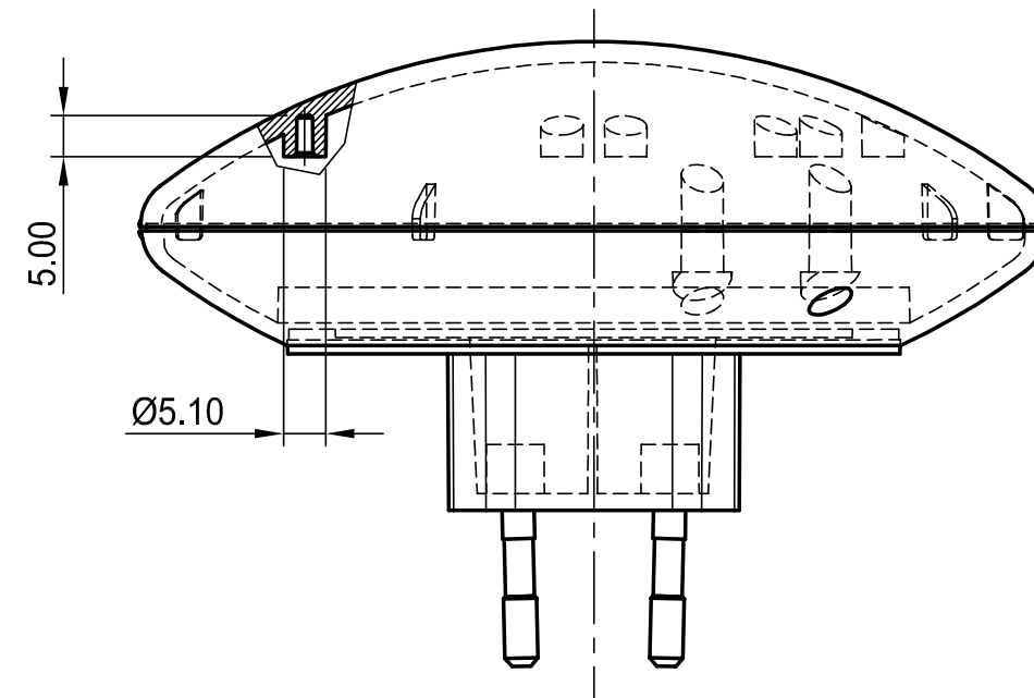
Unterteil- Innenansicht Bottom-Part Inside View
