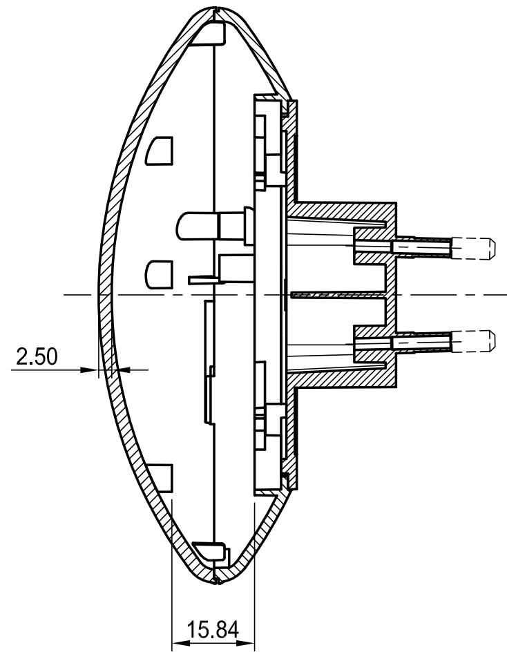
Schnitt A-A section
