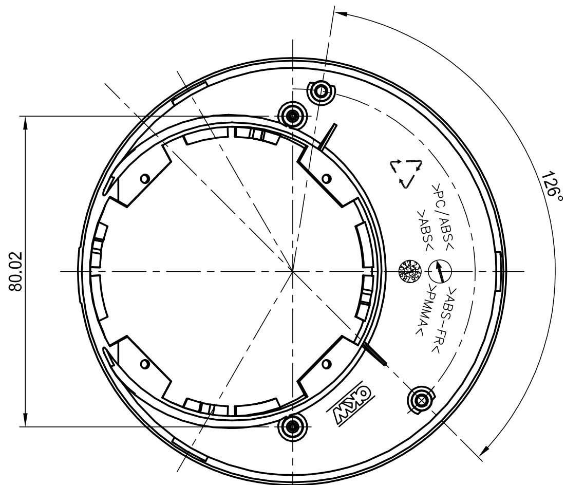
Unterteil- Innenansicht Bottom-Part Inside View
