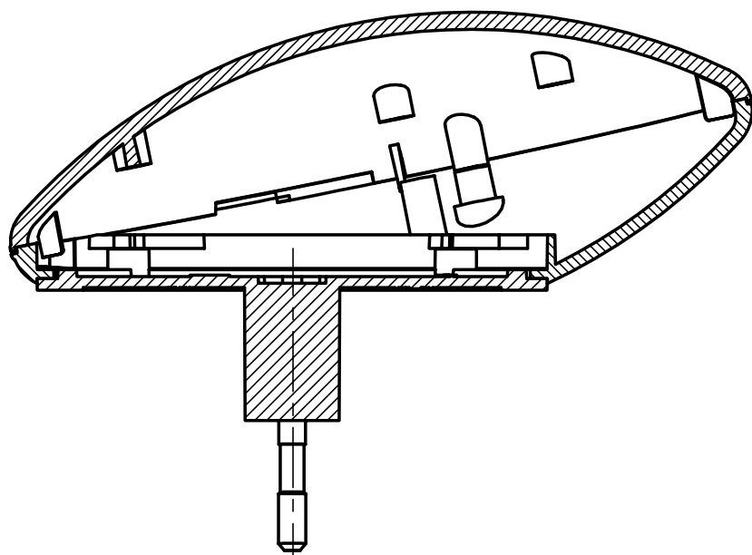
Unterteil- Innenansicht Bottom-Part Inside View
