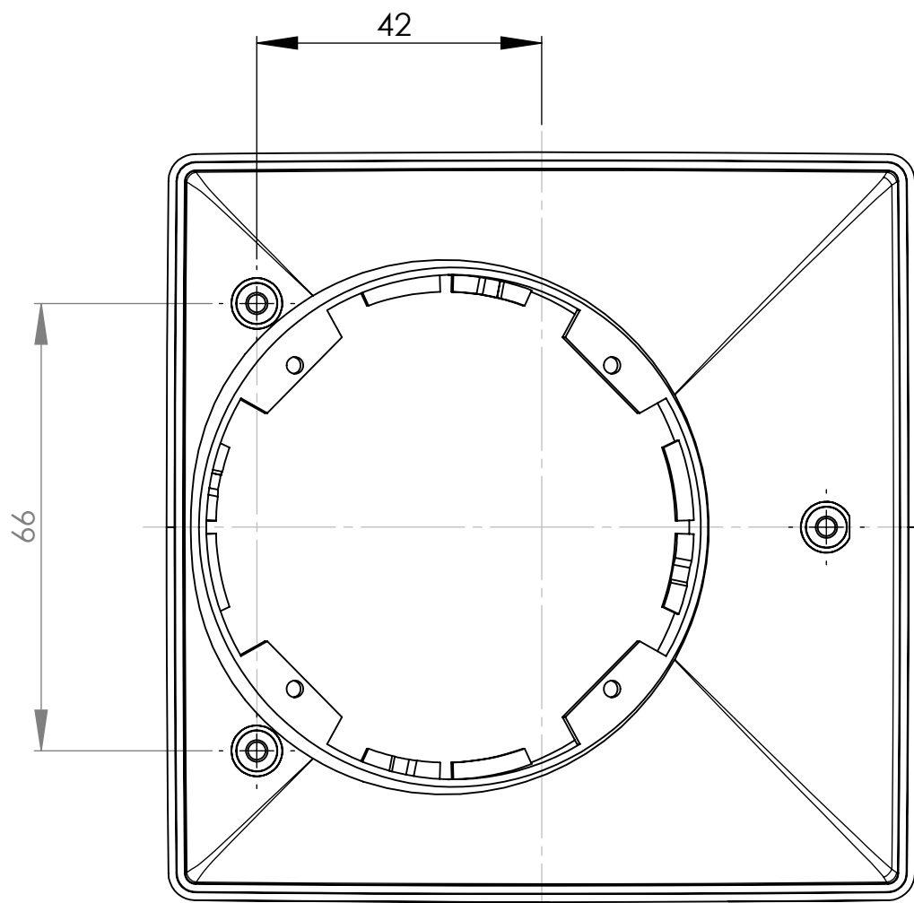
Unterteil-Innenansicht Bottom-Part-Inside-View
