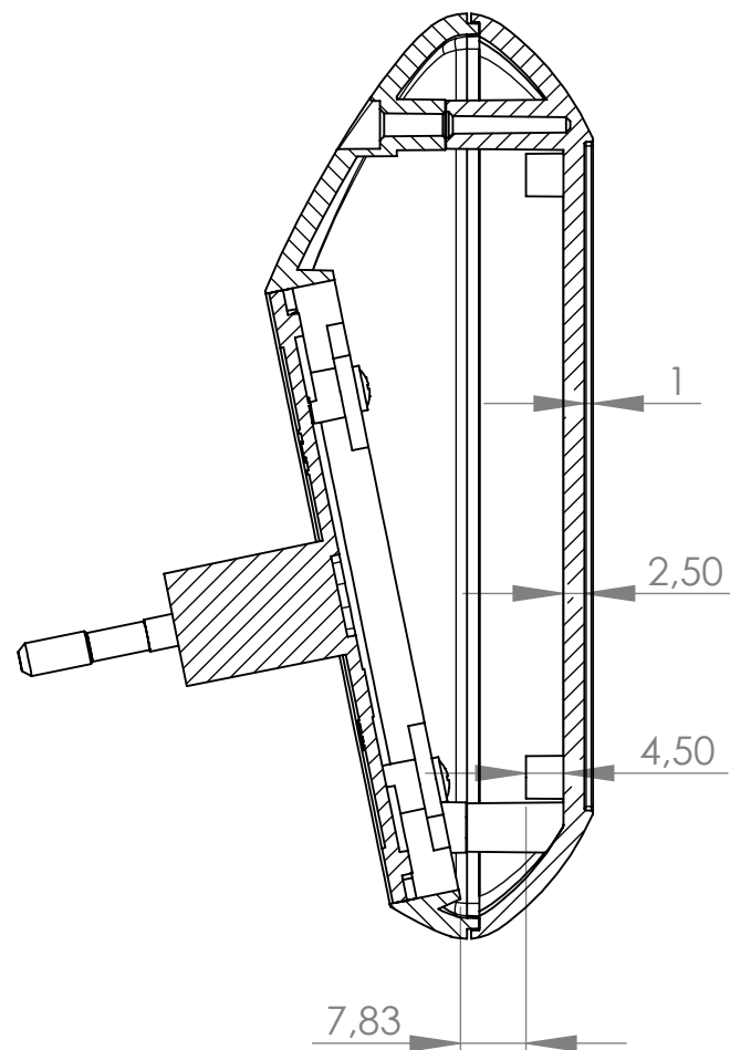
SCHNITT A-A
