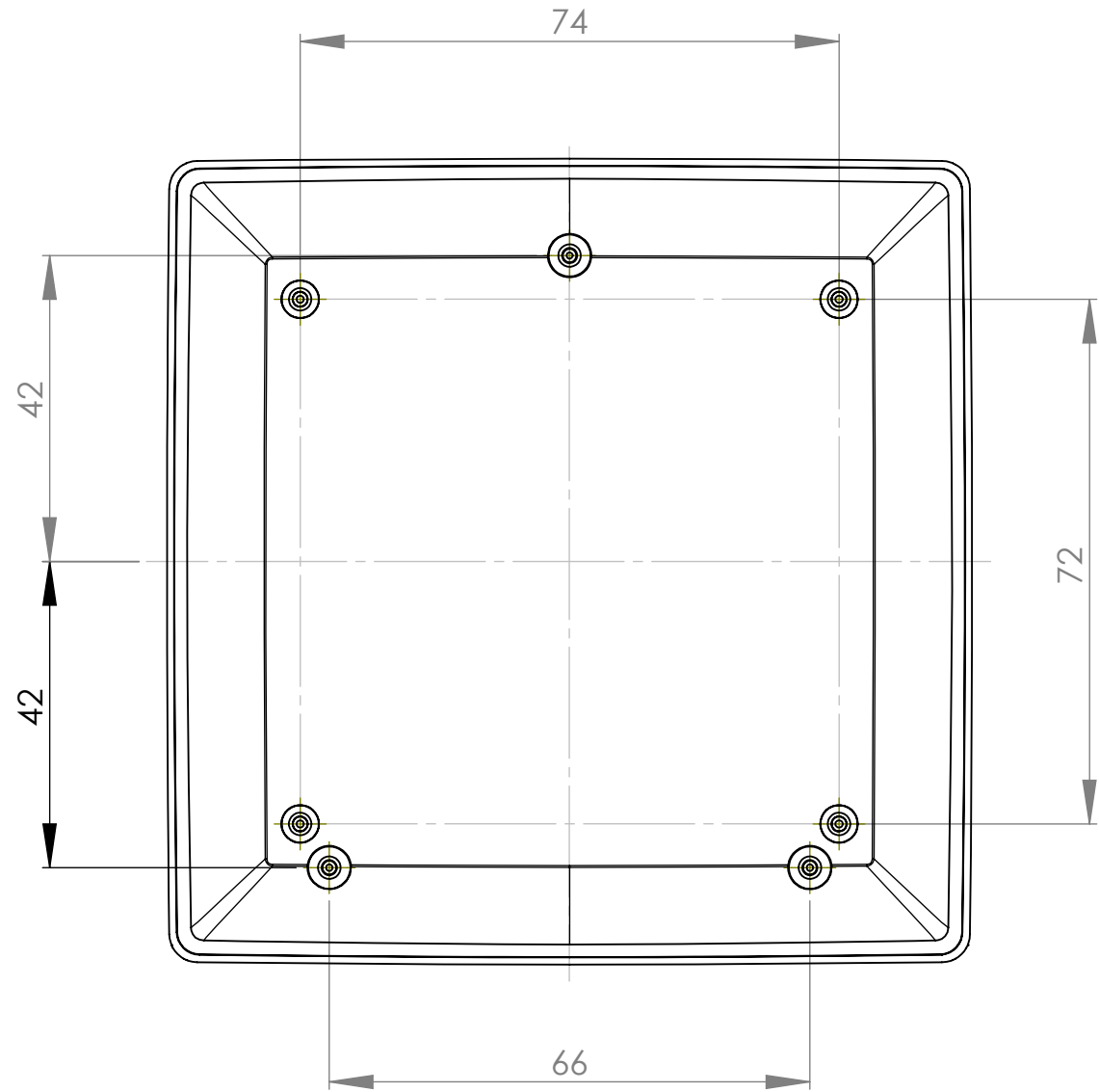
Oberteil-Innenansicht Top-Part-Inside-View
