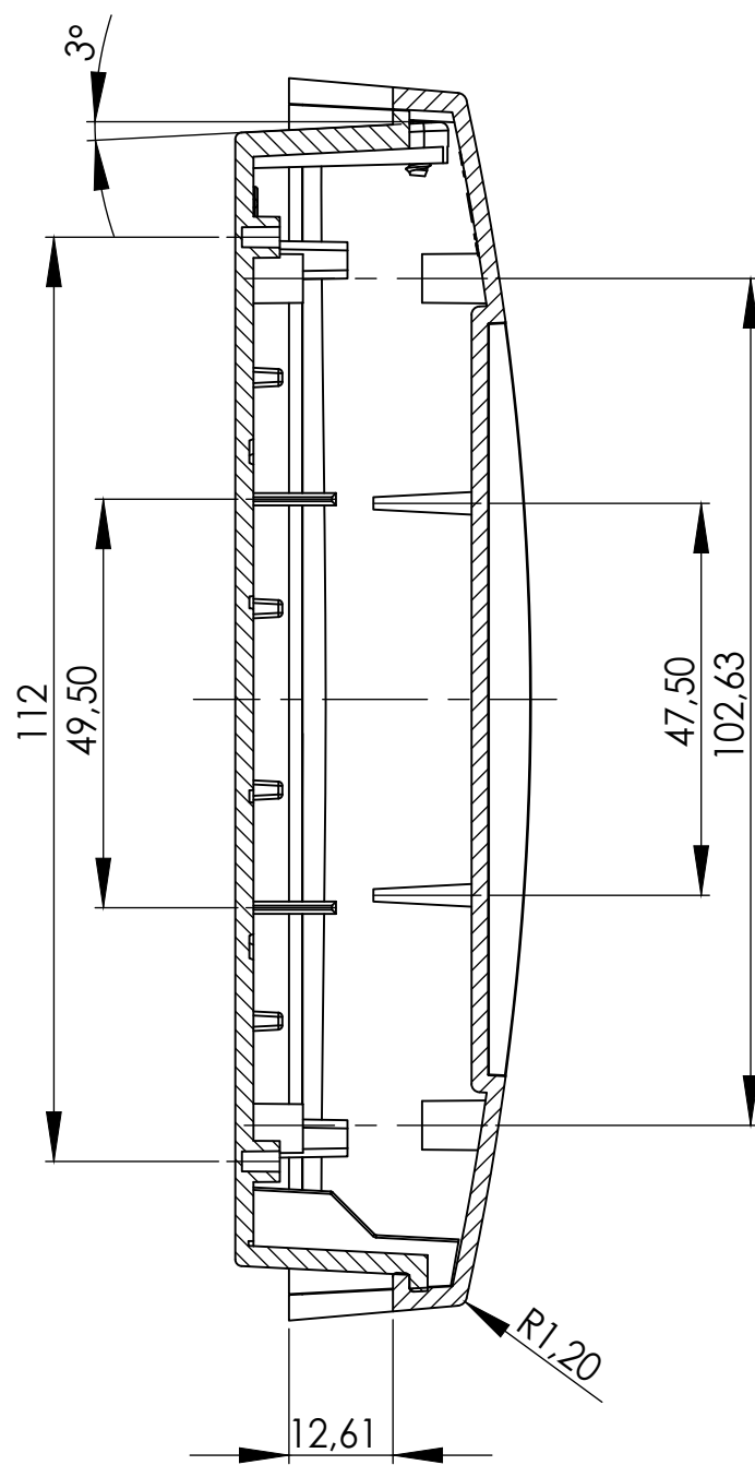
Schnitt A-A
