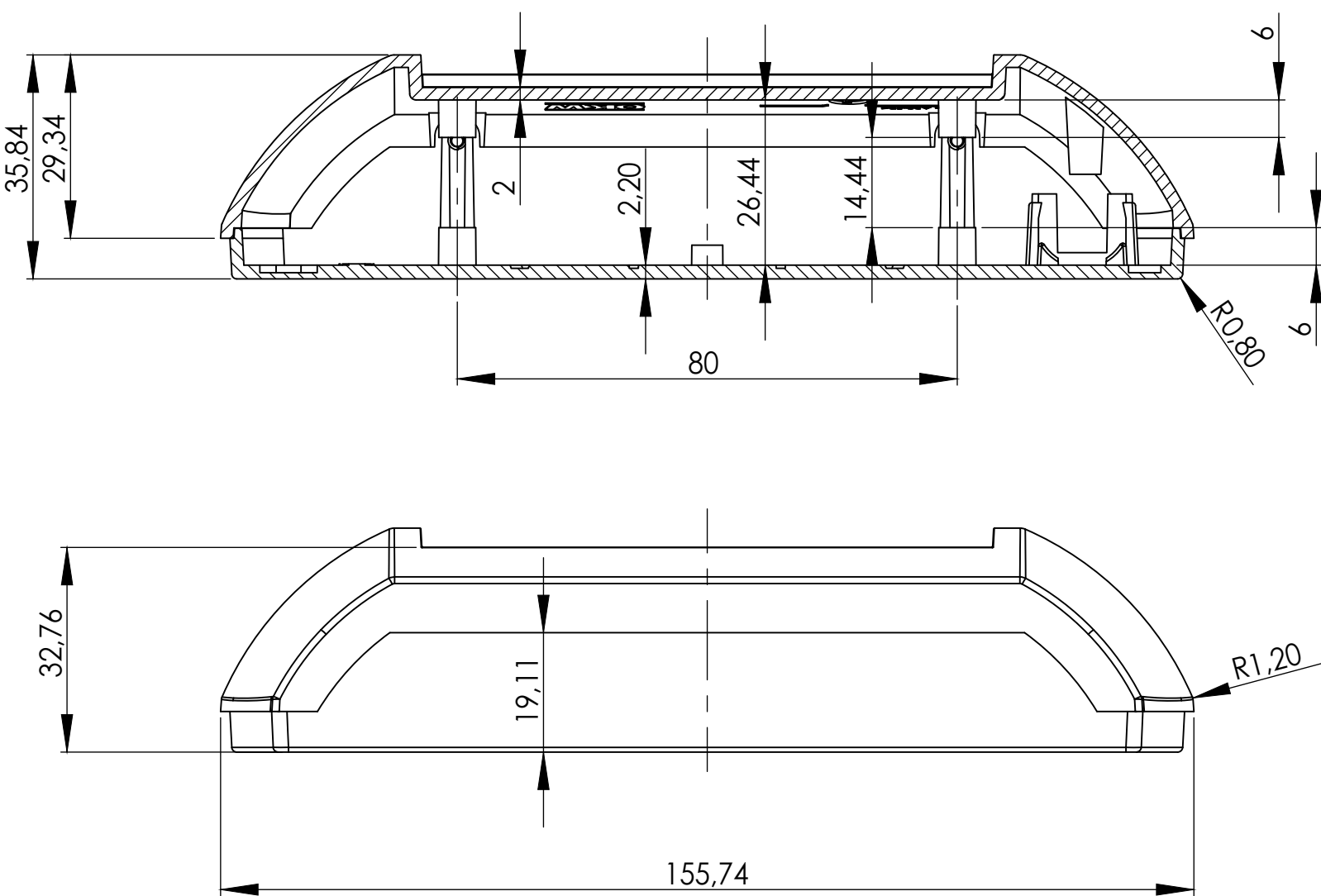
Schnitt C-C
