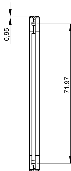
Schnitt A-A
