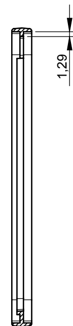
Schnitt B-B
