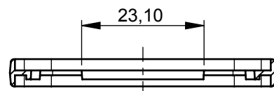
Schnitt C-C
