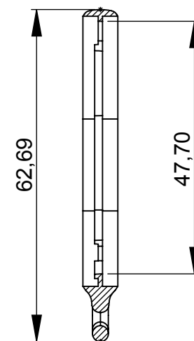
Schnitt A-A
