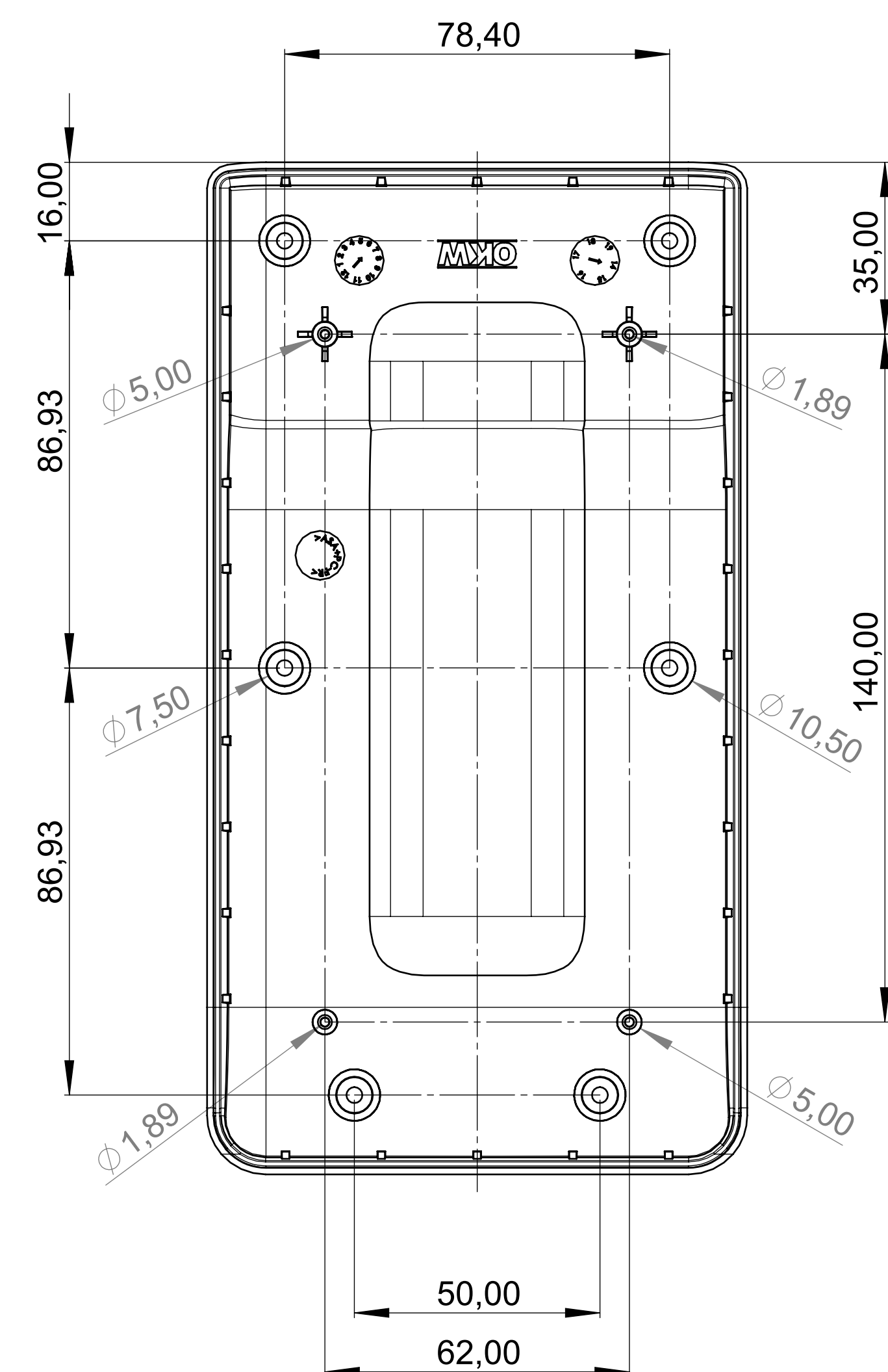
Unterteil Bottom-Part
