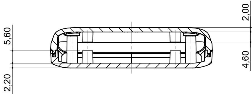
Schnitt B-B
