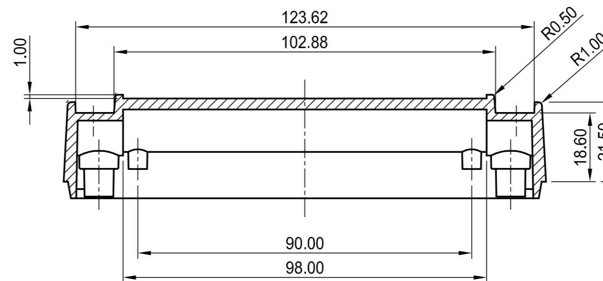
SCHNITT B-B section
