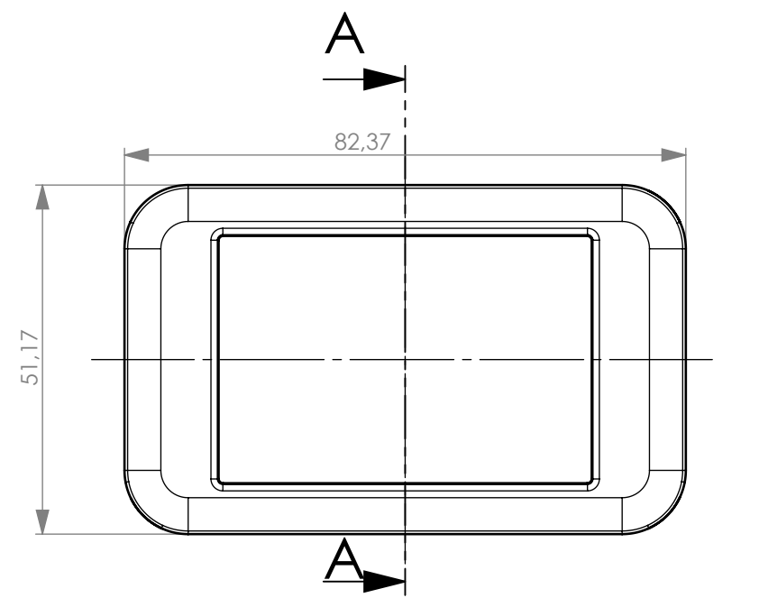
Oberteil Top-Part
