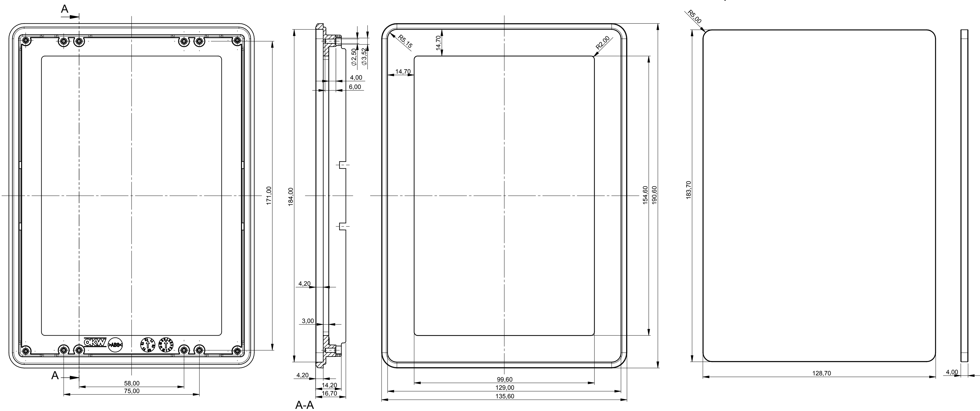
Montageplatte für Glaspanel Mounting plate for glass panel
