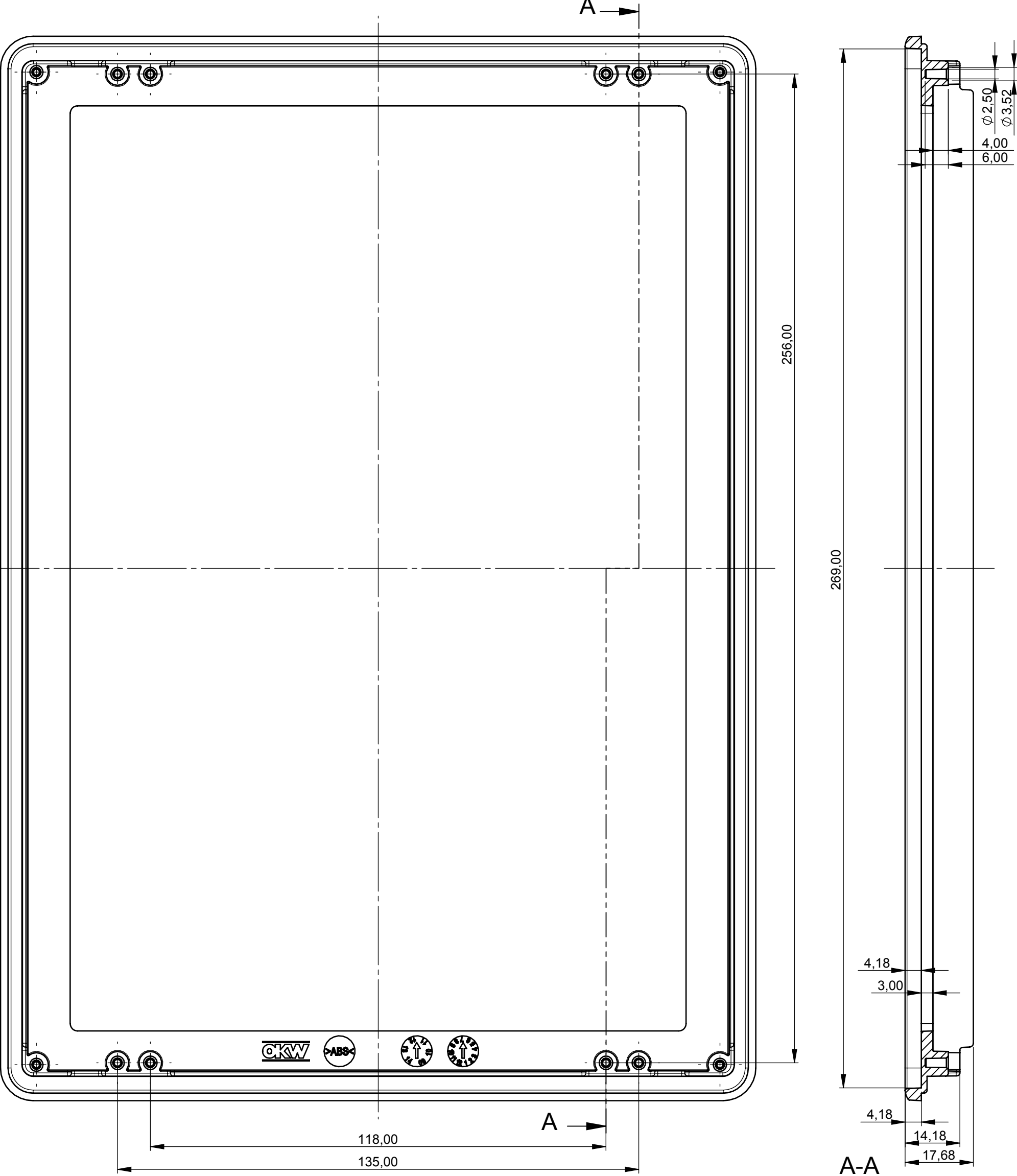
Montageplatte für Glaspanel Mounting plate for glass panel
