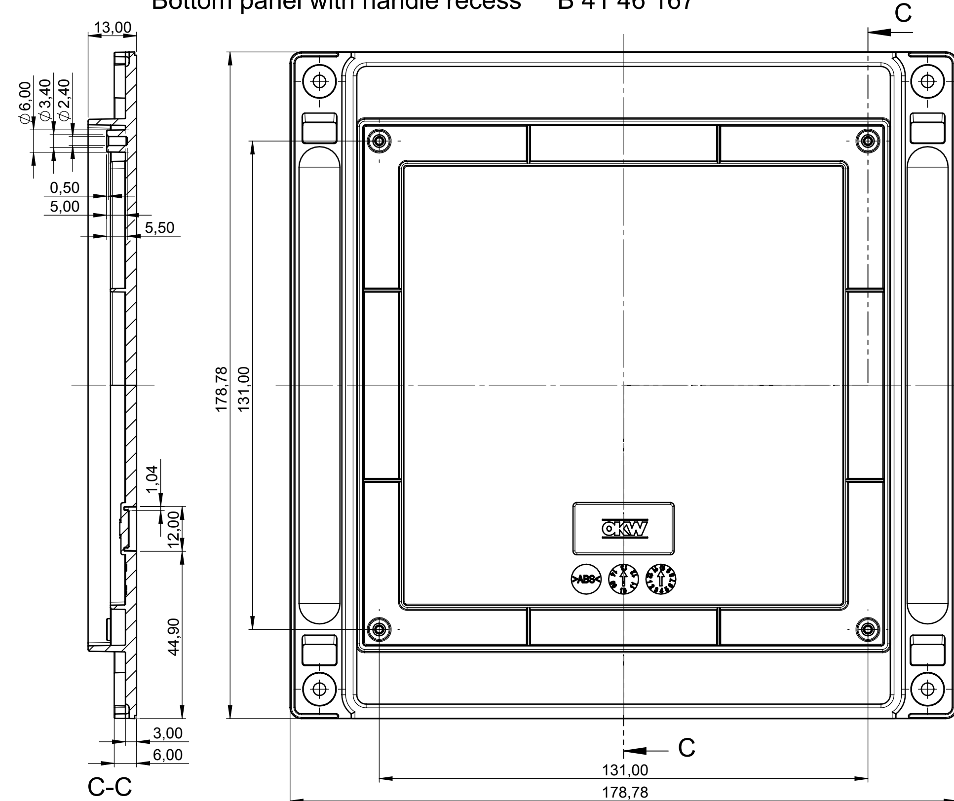
Bodenplatte mit Griffmulde Bottom panel with handle recess B 41 46 167
