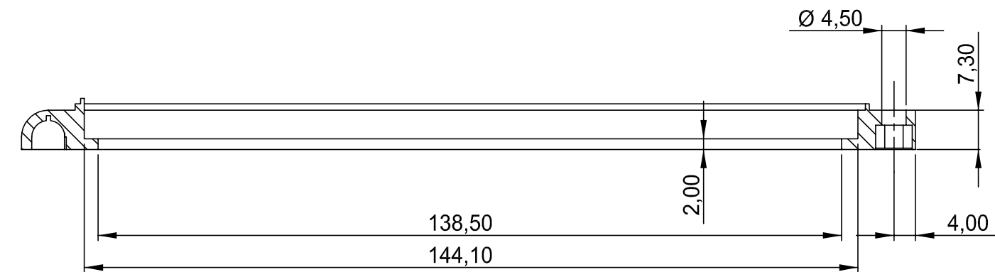
B-B
