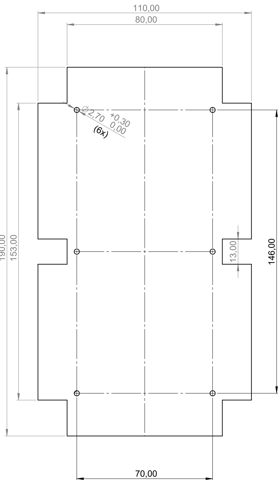
Platine Unterteil P C B Bottom Part
